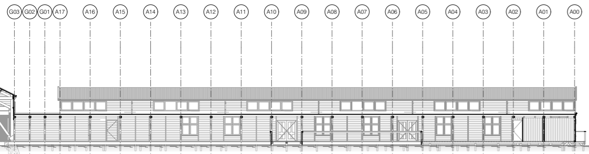
LANGSDOORSNEDE, SCHIP I
