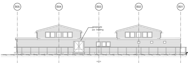
NOORD GEVEL, SCHIP I
