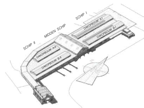
ISOMETRIE
