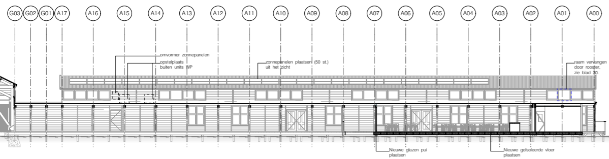
LANGSDOORSNEDE, SCHIP I
