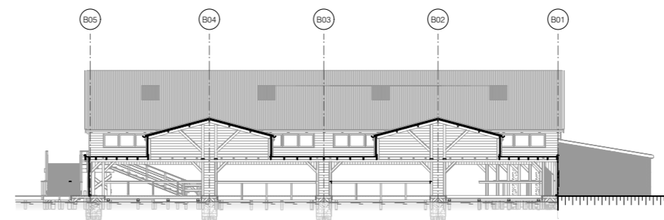
DWARSDOORSNEDE, SCHIP I
