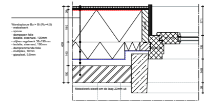
Detailering van de Grote Markt 15
