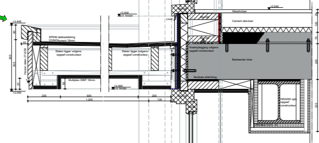
D07: Luifel aansluiting / rand
