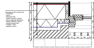
D09: Zijstijl, begane grond
