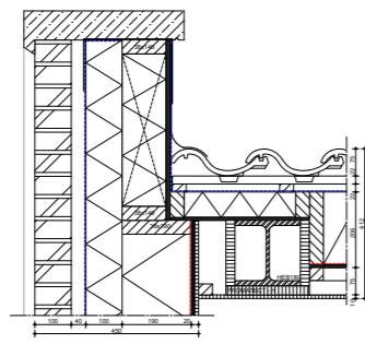
D08: Luifel, dwarsdoorsnede
