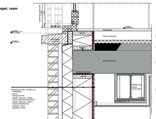
D06: Bovendorpel, raam
