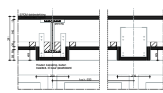
D05: Zijstijl, tweede verdieping
