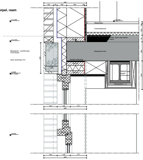
D04: Onderdropel, raam
