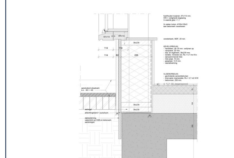
Afbeelding 6, 7, 8. Linksonder: dwarsdoorsnede met links de belending en rechts de gevel aan het kerkplein voor de Laurentiuskerk. Linksonder: horizontaal detail met zinken bekleding tegen de steunbeer van de Laurentiuskerk, verspringende smalle en brede kozijnen, dubbele kolommen en de vooruitspringende entree. Rechts: verticale details van de luifel met daarboven zinken gevelbekleding met luifel en plafond op zelfde hoogte en onderdetail van het kozijn met brede vensterbank op een hardstenen plint 2025.
