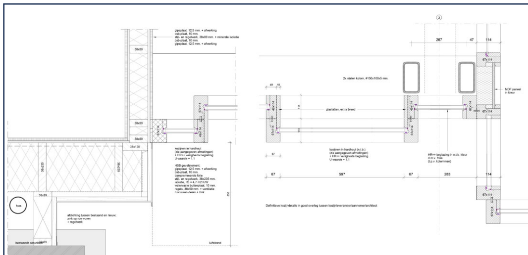
Afbeelding 6, 7, 8. Linksonder: dwarsdoorsnede met links de belending en rechts de gevel aan het kerkplein voor de Laurentiuskerk. Linksonder: horizontaal detail met zinken bekleding tegen de steunbeer van de Laurentiuskerk, verspringende smalle en brede kozijnen, dubbele kolommen en de vooruitspringende entree. Rechts: verticale details van de luifel met daarboven zinken gevelbekleding met luifel en plafond op zelfde hoogte en onderdetail van het kozijn met brede vensterbank op een hardstenen plint 2025.
