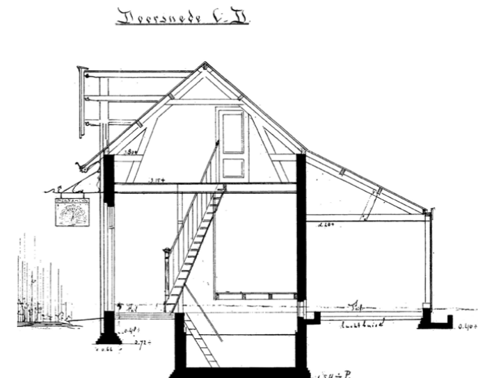
Oorspronkelijke bouwtekeningen J.J. van Wort, vooraanzicht en doorsnede met kelder
