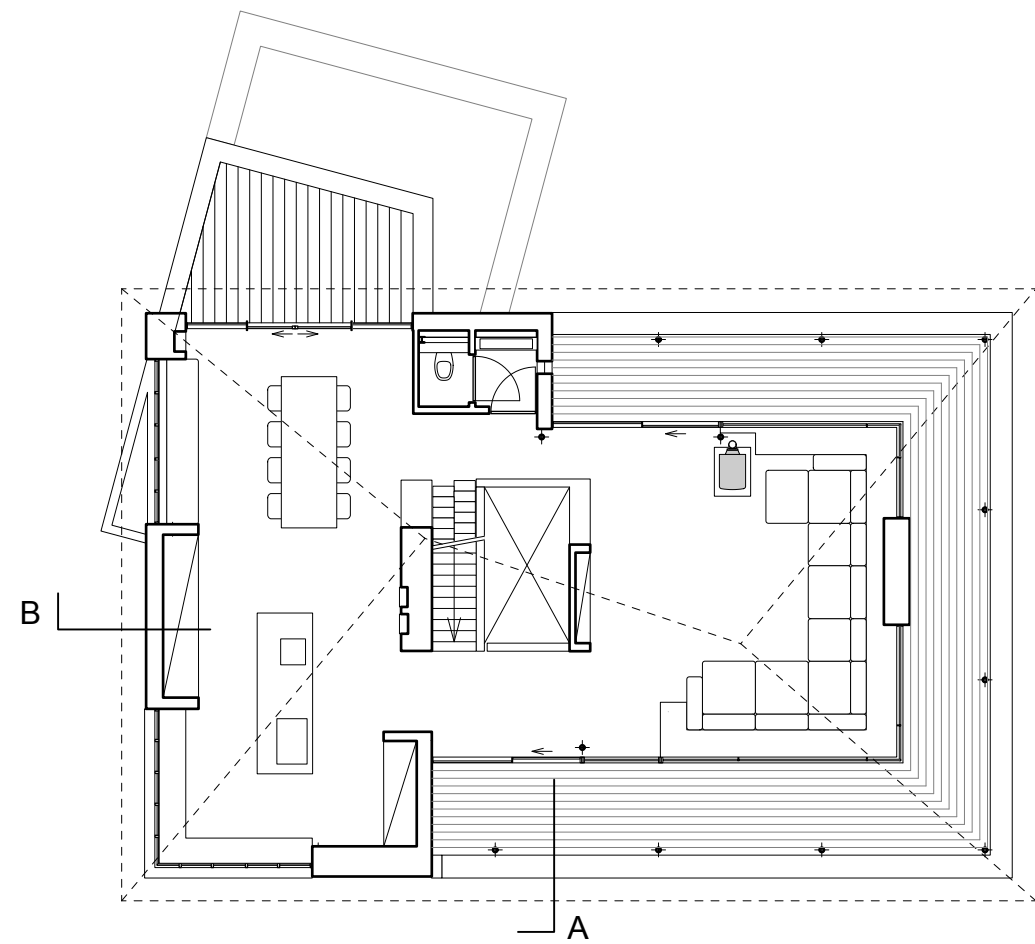
1e VERDIEPING
