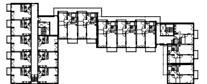
typische plattegrond
