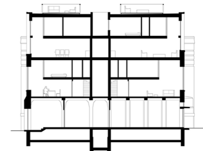
standaard doorsnede
