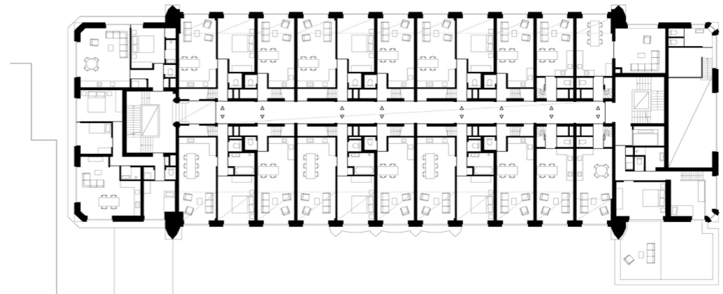
eerste verdieping
