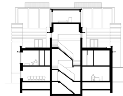
doorsnede trappenhuis
