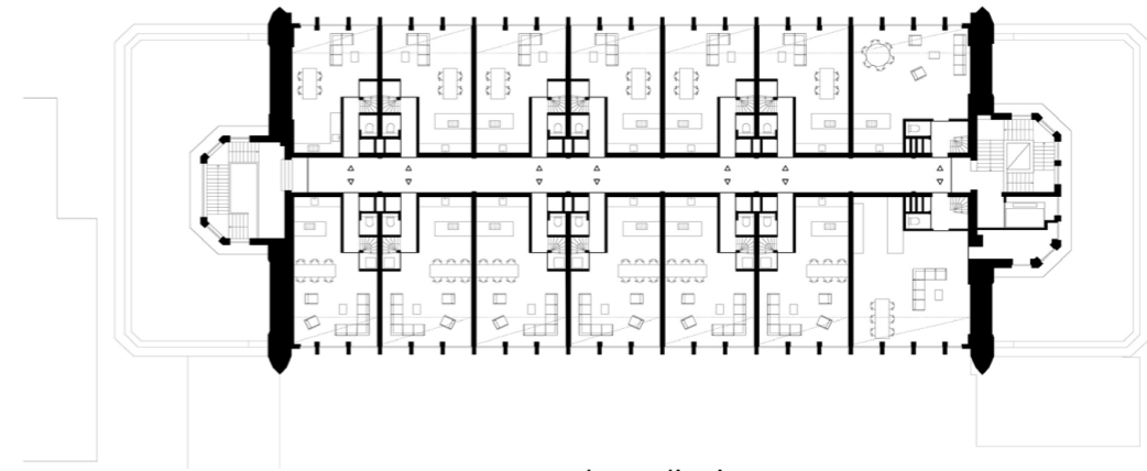
tweede verdieping
